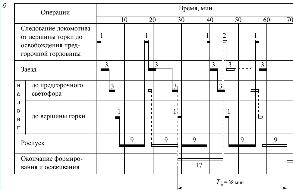
Рис. 2.25. Технологический график работы горки при двух горочных локомотивах
