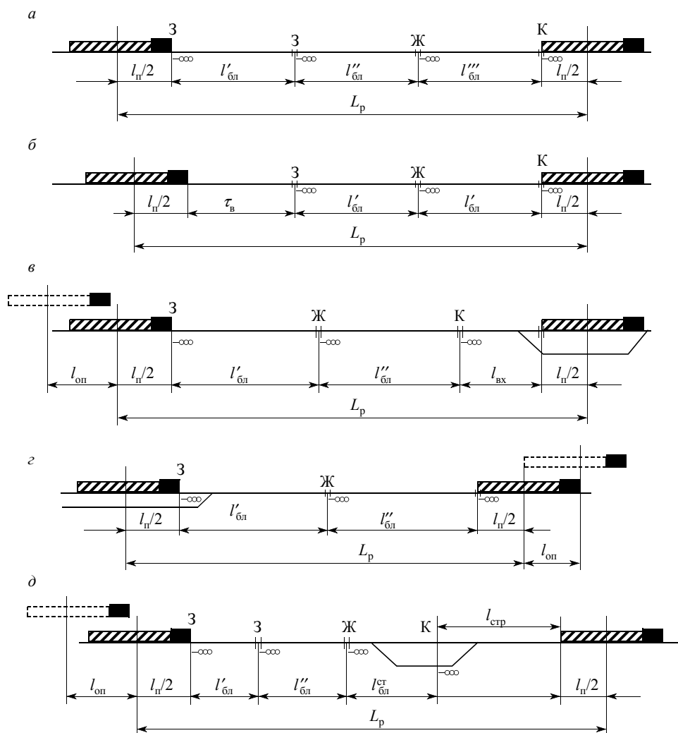
Рис. 5.20. Схемы расположения поездов, следующих в пакете при автоблокировке: a, б — разграничение поездов тремя и двумя блок-участками; в — разграничение поездов при приеме на станцию; г — разграничение поездов при отправлении на станции; д — разграничение поездов при безостановочном пропуске через станцию; К, Ж, 3 — красный, желтый и зеленый огни светофора
