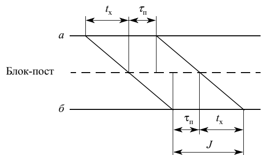
Рис. 5.22. Интервал в пакете при полуавтоматической блокировке
