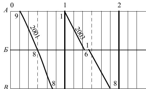
Рис. 5.2. Линии хода поездов на графике движения
