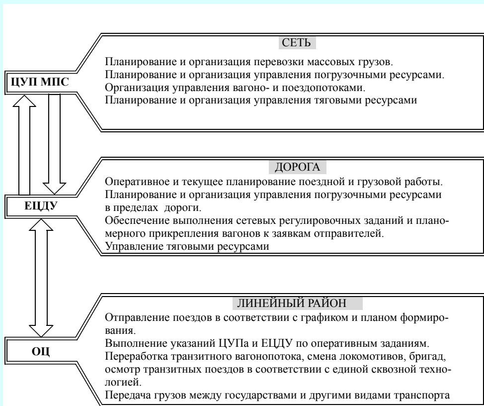
Рис. 1.1. Схема сети центров управления перевозками
