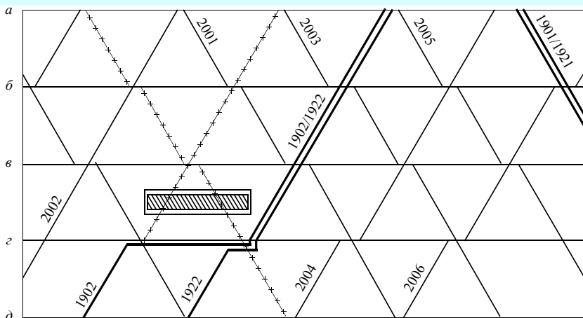
Рис. 5.43. Схема пропуска двояных поездов на однопутной линии при выделении «окна»
