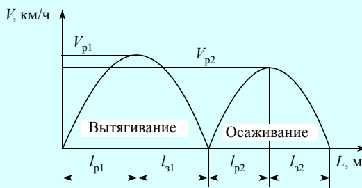
Рис. 2.7. Диаграмма изменения скорости при выполнении полурейсов:
